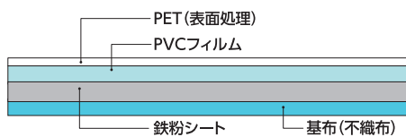
製品構成 拡大図
